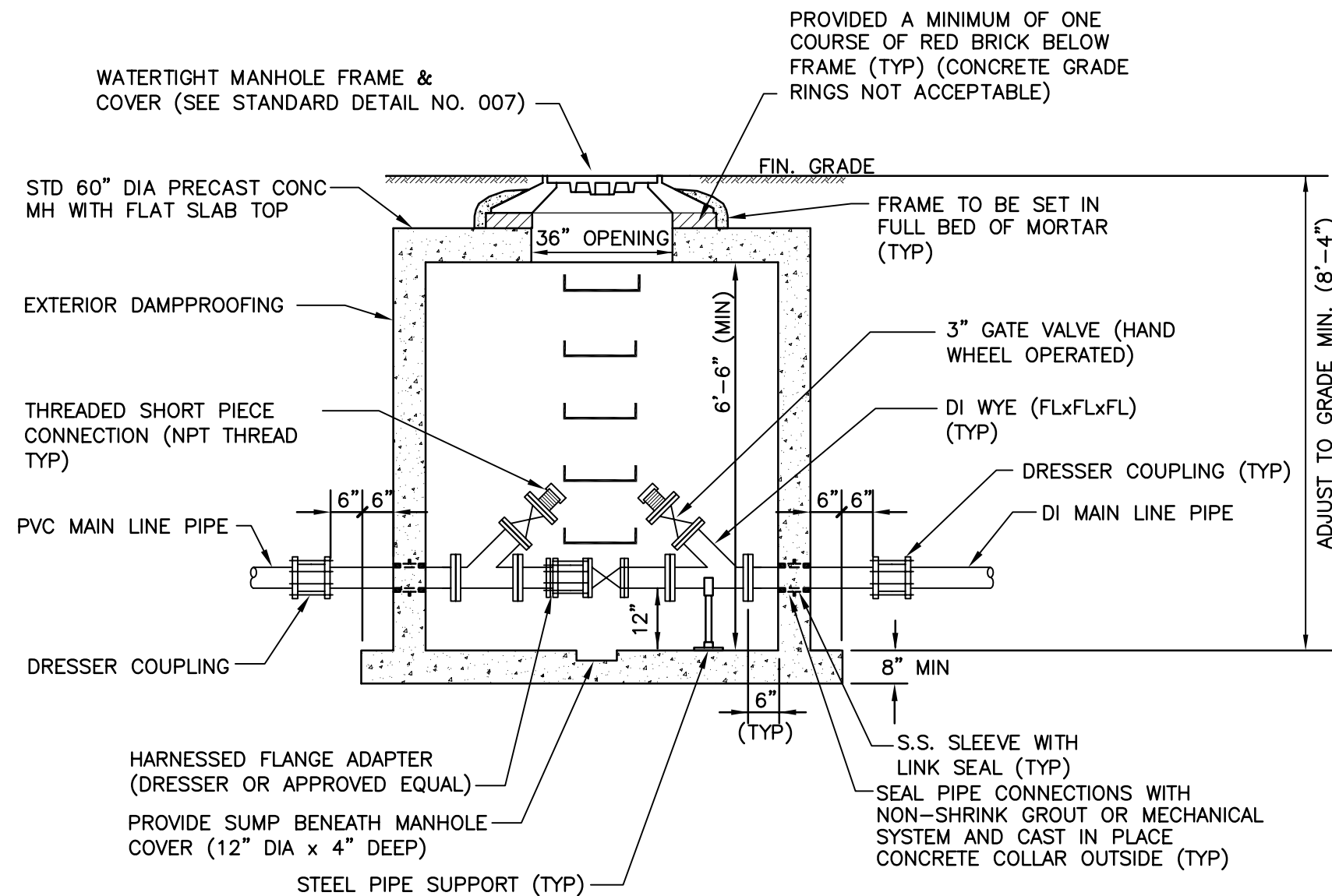
SECTION A-A
